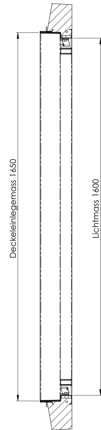
SCHNITT A-A MABSTAB 1 : 8
